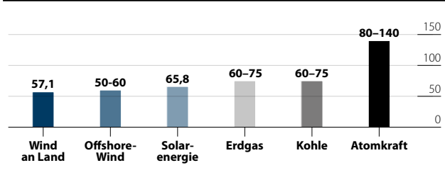
Daten: Öko-Institut Freiburg: Kosten neuer Stromerzeugungsanlagen, August 2017
